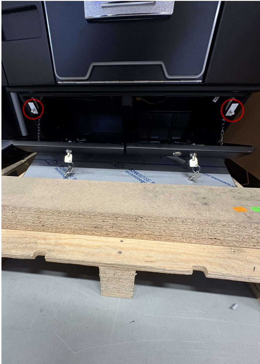
Türschalter der linken und rechten Wartungsklappe
