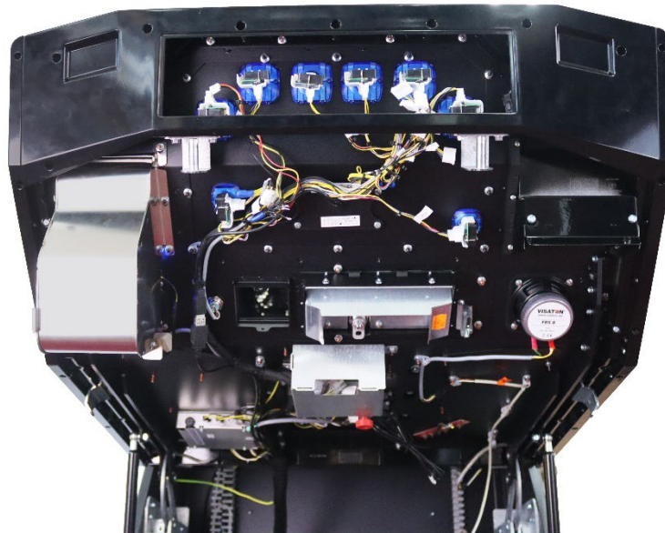
ELT-000777-01 Lüfter Ausgang, 2x Ersatz Ausgang
